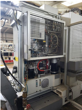
Späneförderer
