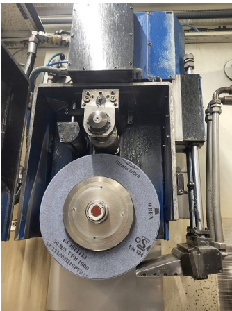
Schleifscheibe
